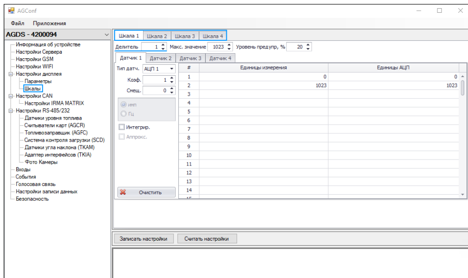
Рис.57. Настройка простой шкалы.
