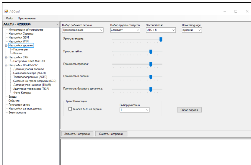
Рис.25. Настройка основных параметров устройства.
