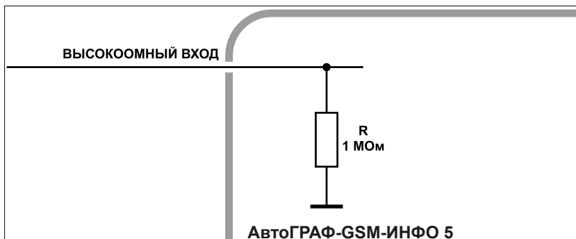
Рис.111. Внутренняя схема высокоомного входа.
