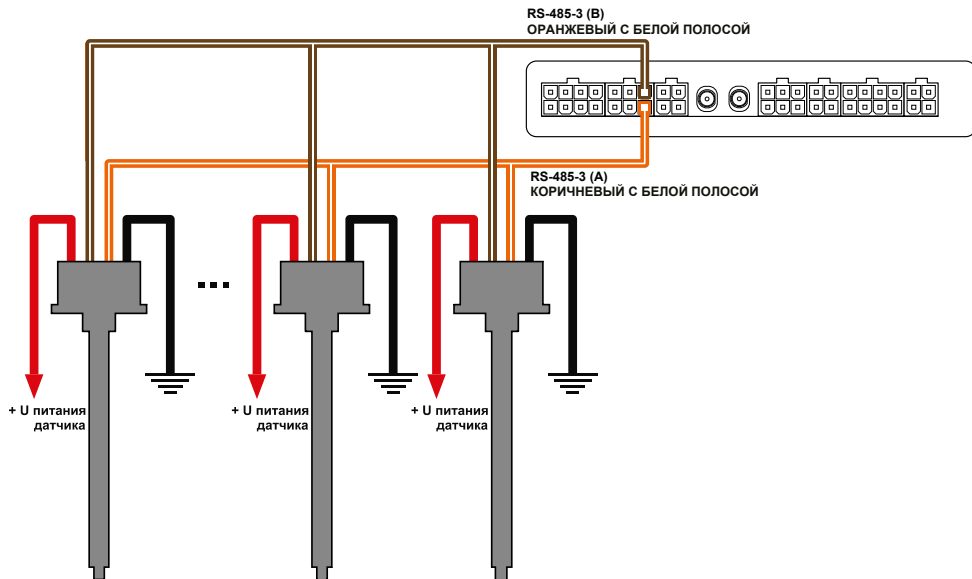
Рис.122. Внутренняя схема подключения датчиков уровня топлива.
