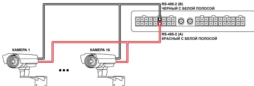
Рис.121. Структурная схема подключения камер.
