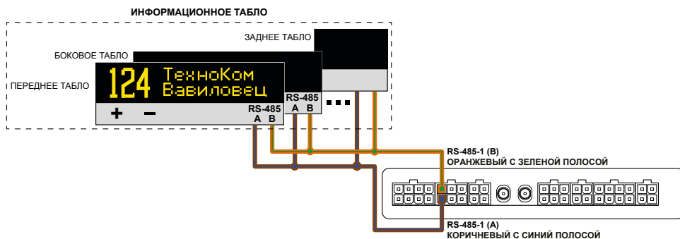
Рис.118. Структурная схема подключения информационных табло.
