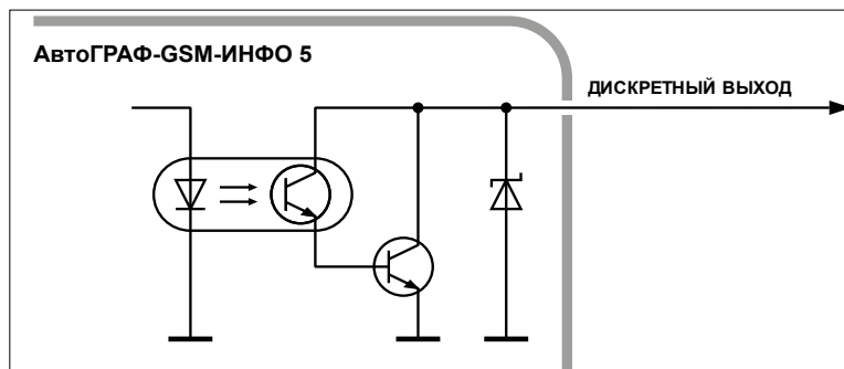
Рис.115. Внутренняя схема цифрового выхода.
