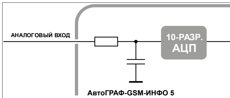
Рис.114. Внутренняя схема аналогового входа.
