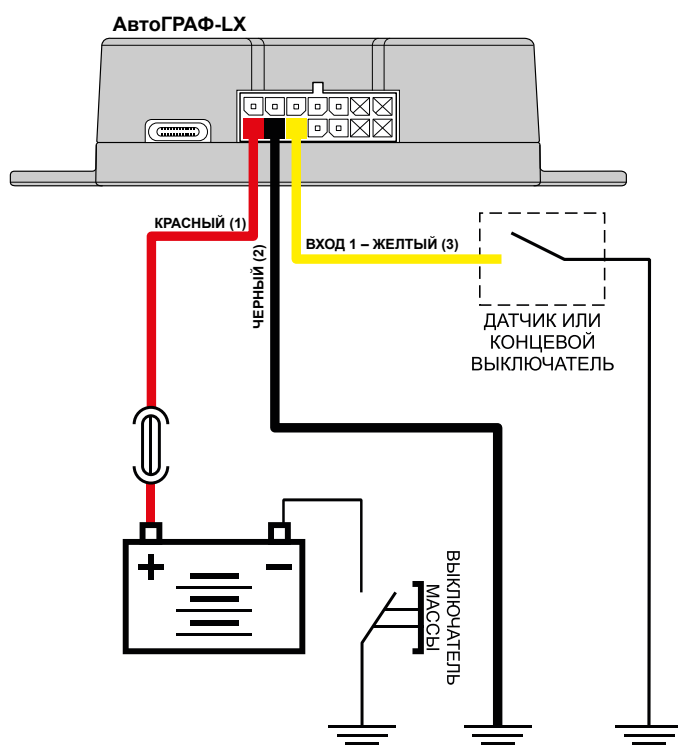
2 – с подтяжкой, подключение питания после выключателя массы
