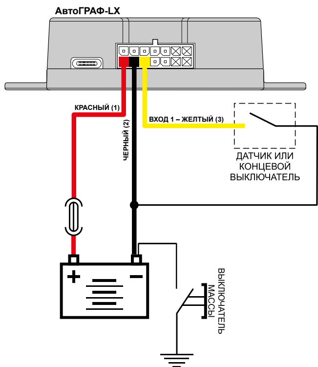
1 – с подтяжкой, подключение питания до выключателя массы
